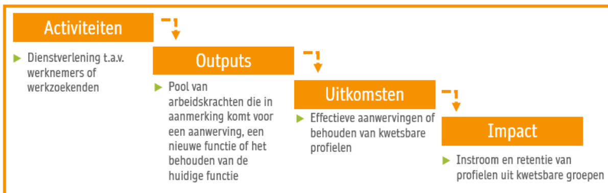
Figuur 25: Resultatenketen 2
